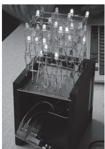
LED-Cube bauen und programmieren
